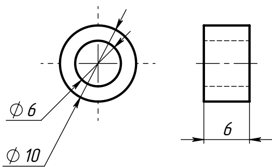
Поз.3 (Втулка) паронит 2 : 1
