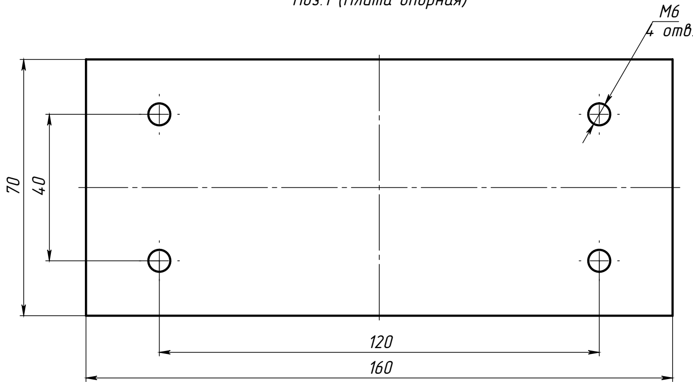
Поз.1 (Плита опорная)
