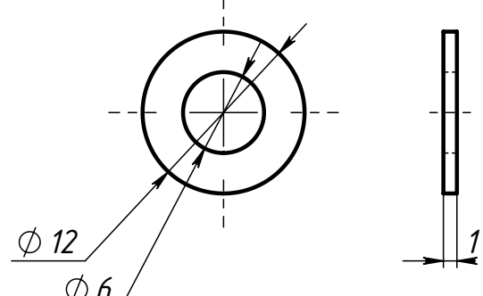
Поз.4 (Шайба) паронит 2 : 1
